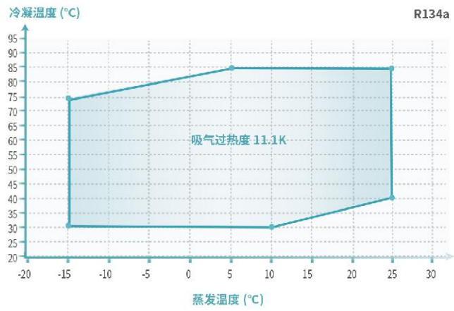
序号 1-6 产品型号: 适用此运行范围图
